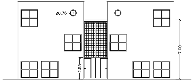
PROSPETTO PRINCIPALE
