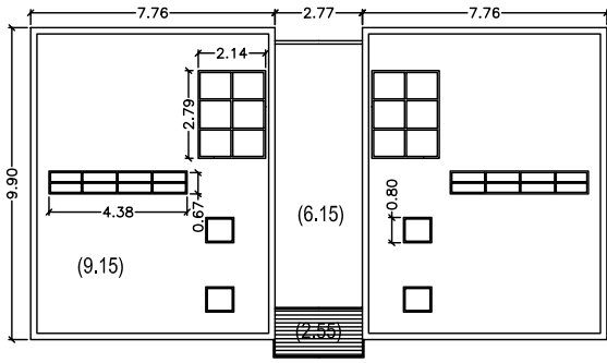
PIANTA COPERTURE
