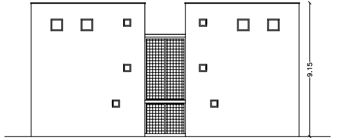
PROSPETTO POSTERIORE
