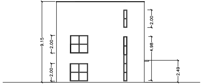
PROSPETTO LATERALE
