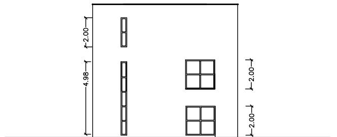
PROSPETTO LATERALE
